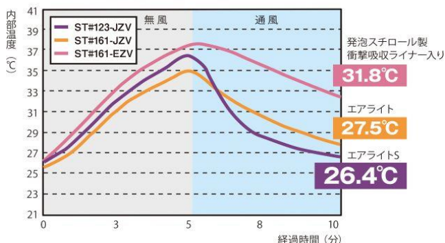
通風による帽体内部の温度比較*
